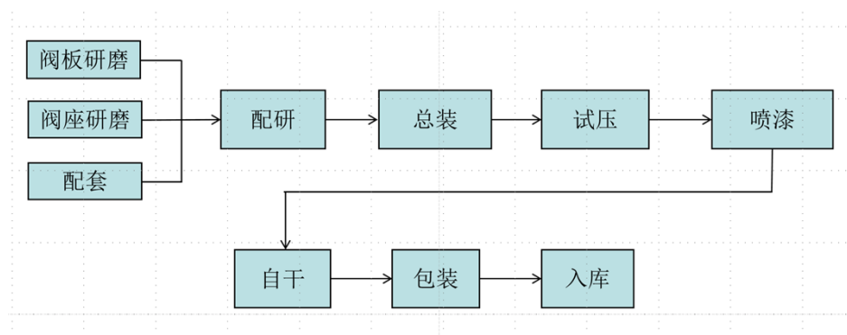
受核查方生产工艺流程图
